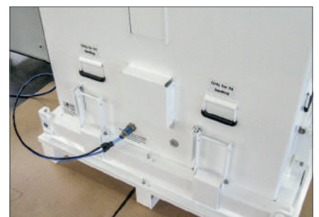
Wasserdampfdichter Behälter bei Dichtheitsprüfung durch Überdruck
