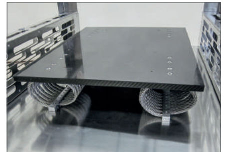
Aufnahmefähig, schwingend gelagert mit Gummipuffer oder Drahtseildämpfer
